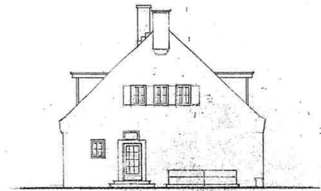
FIG.8. R. Z'IJGEVEL.
