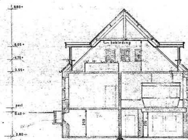
FIG.9. DOORSNEDEN A-B
