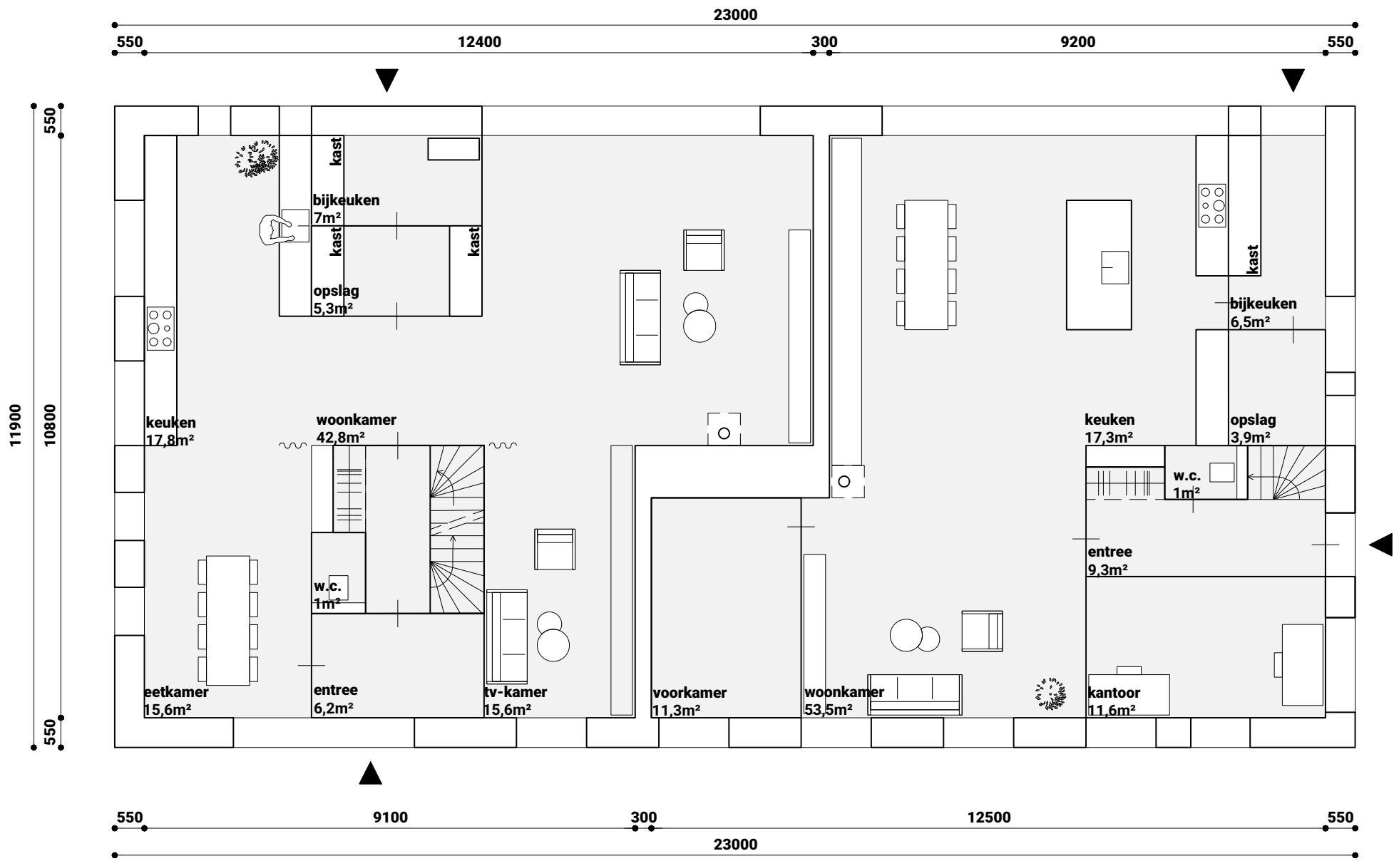
PLATTEGROND BEGANE GROND VARIANT OVERLOOP (SCHAAL 1/100)
