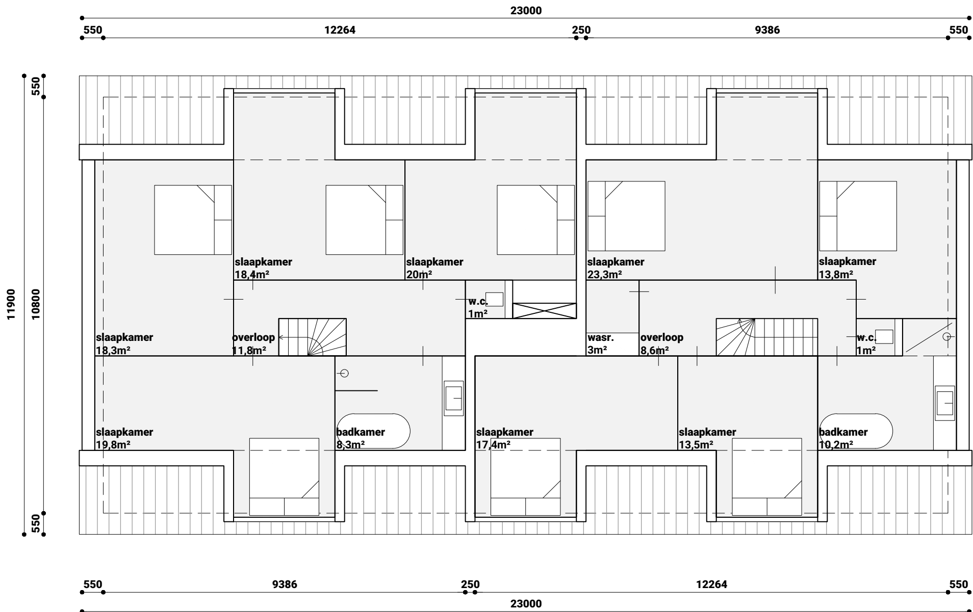
PLATTEGROND VERDIEPING VARIANT OVERLOOP (SCHAAL 1/100)
